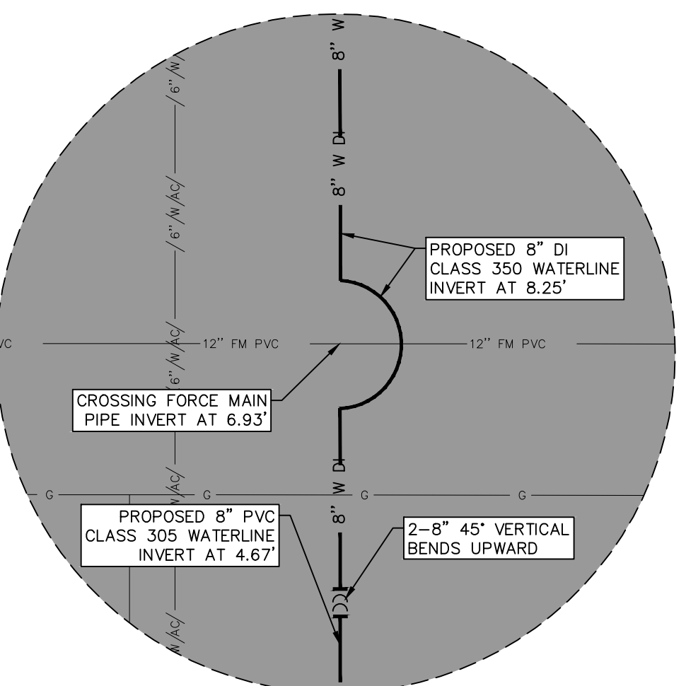
INSET 27 SCALE: 1"=5'
