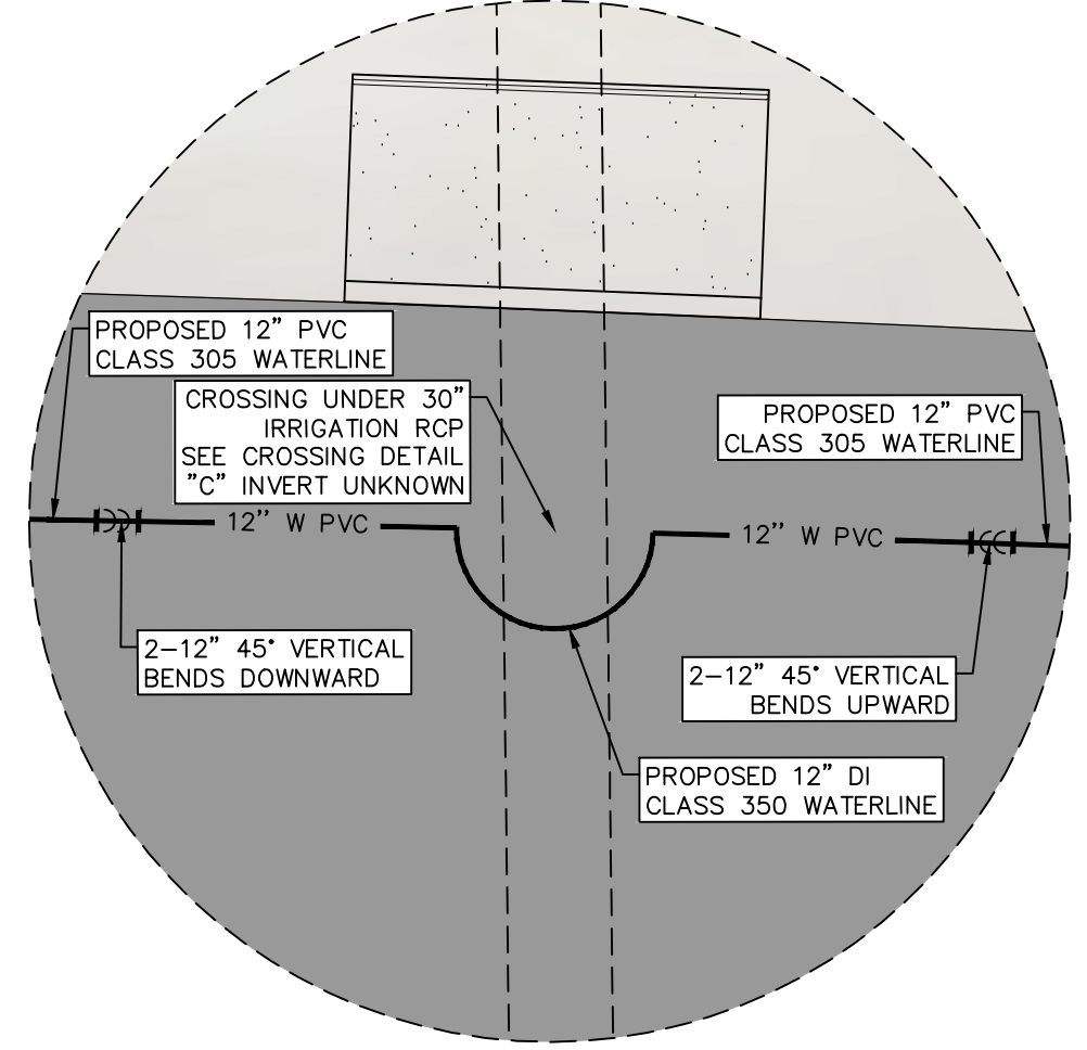
INSET 17 SCALE: 1"=5'
