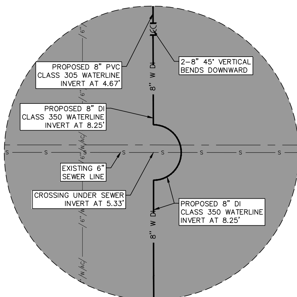
INSET 26 SCALE: 1"=5'
