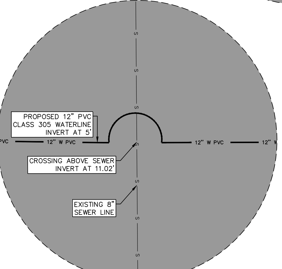
INSET 14 SCALE: 1"=5'
