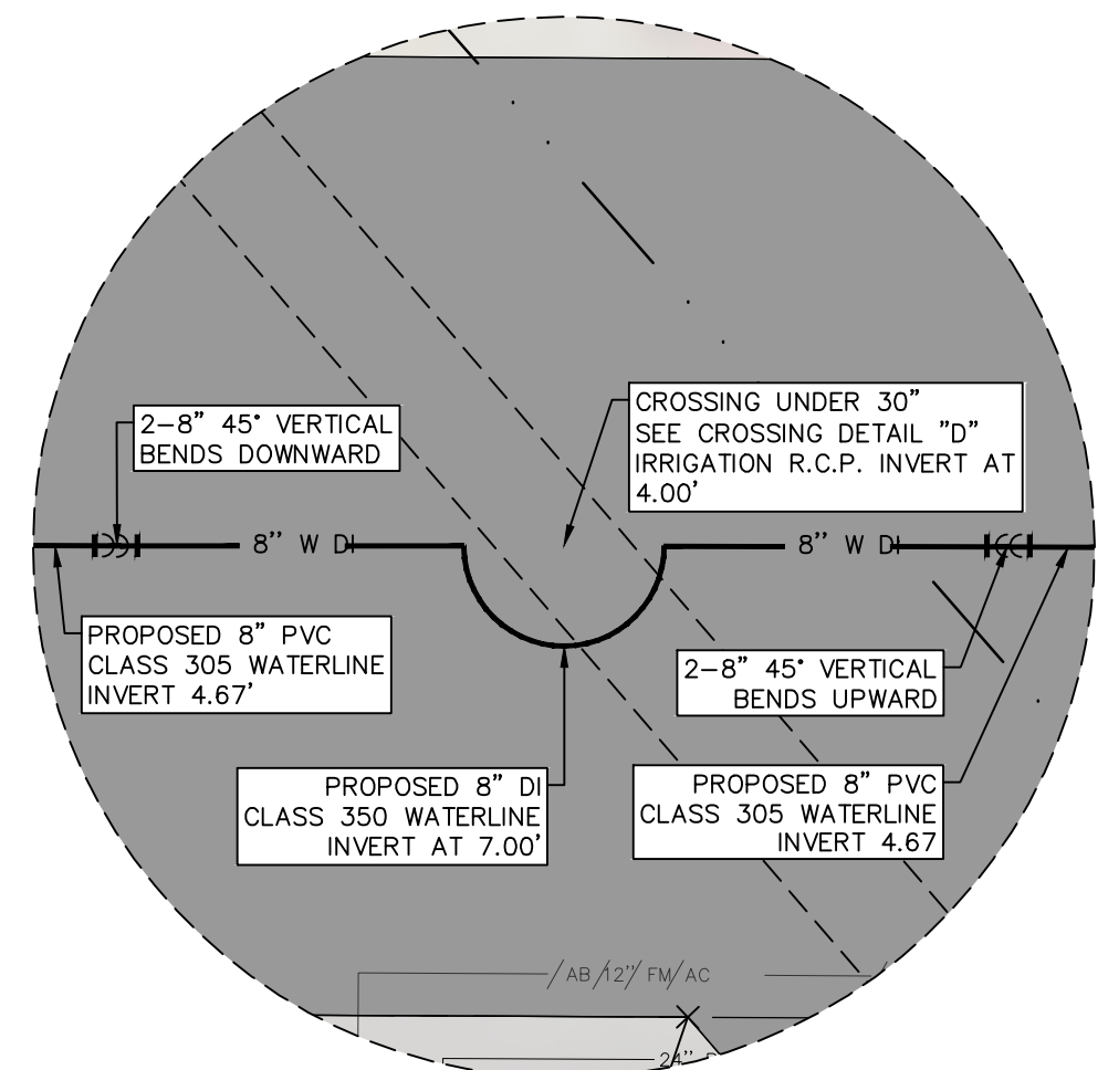
INSET 20 SCALE: 1"=5'
