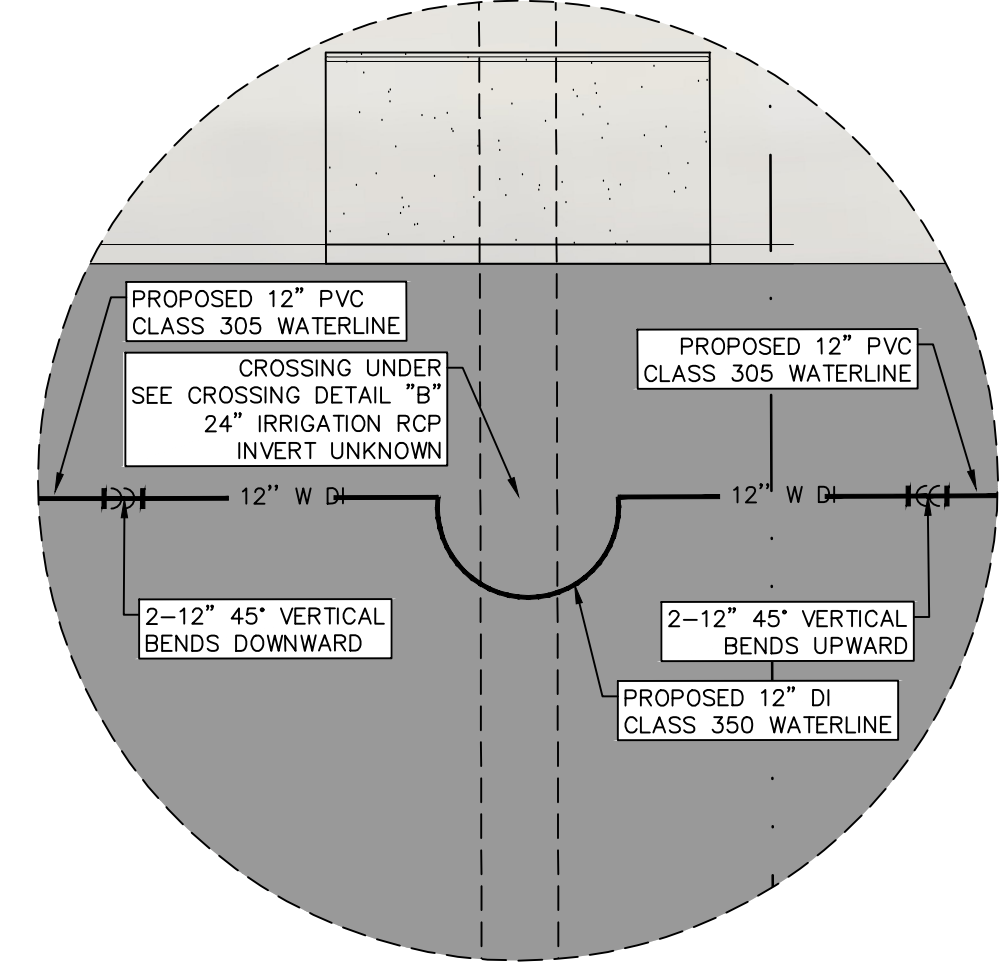
INSET 16 SCALE: 1"=5'
