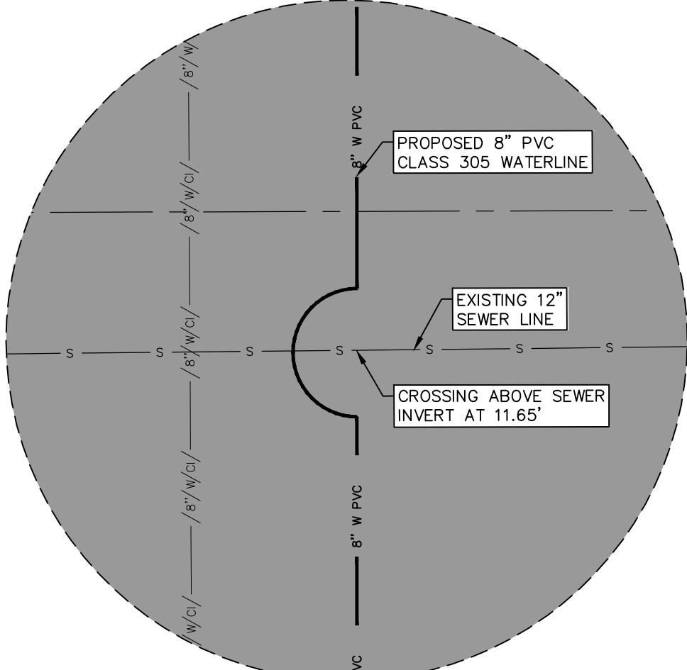
INSET 11 SCALE: 1"=5'
