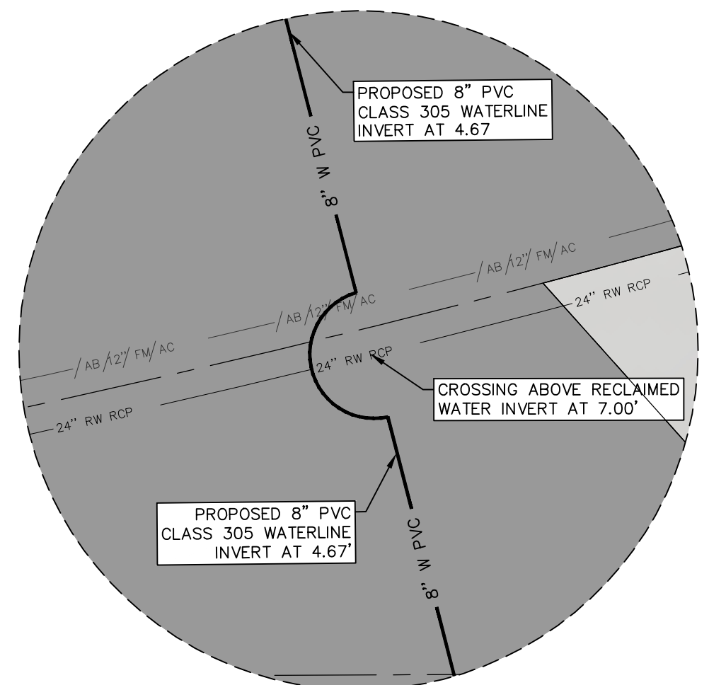
INSET 21 SCALE: 1"=5'
