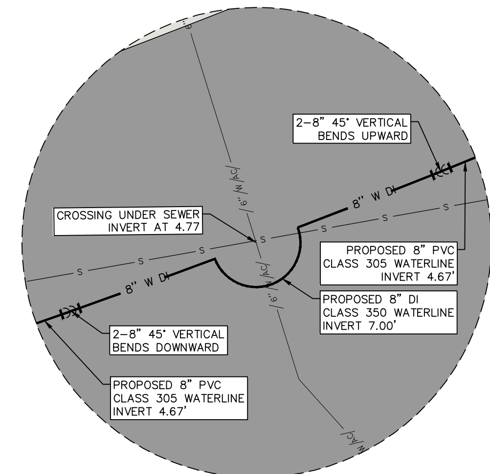
INSET 23 SCALE: 1"=5'
