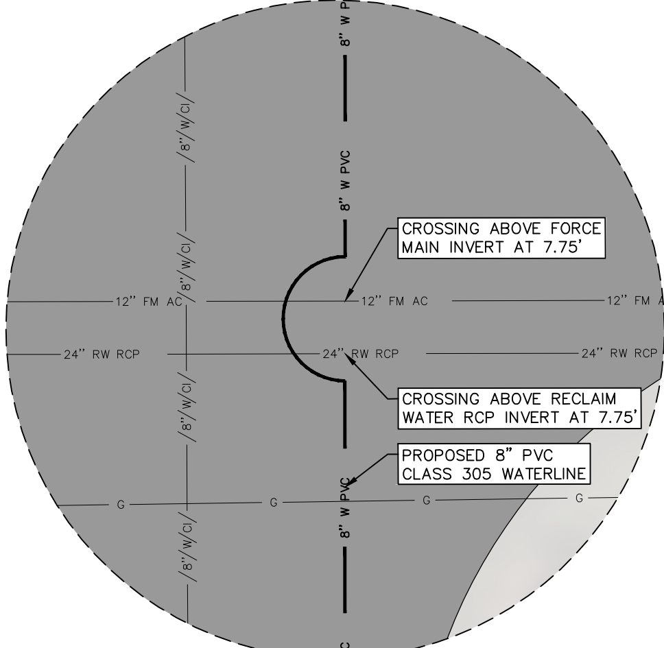
INSET 12 SCALE: 1"=5'
