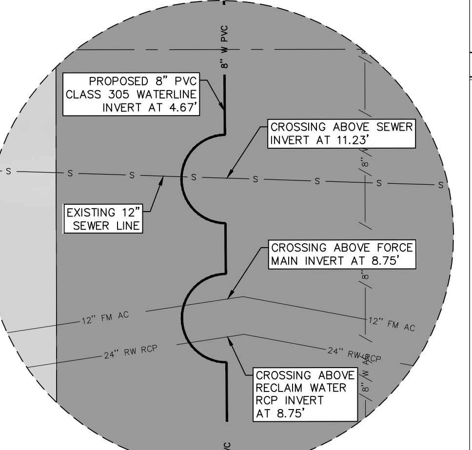
INSET 15 SCALE: 1"=5'
