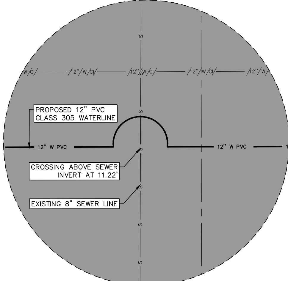
INSET 10 SCALE: 1"=5'
