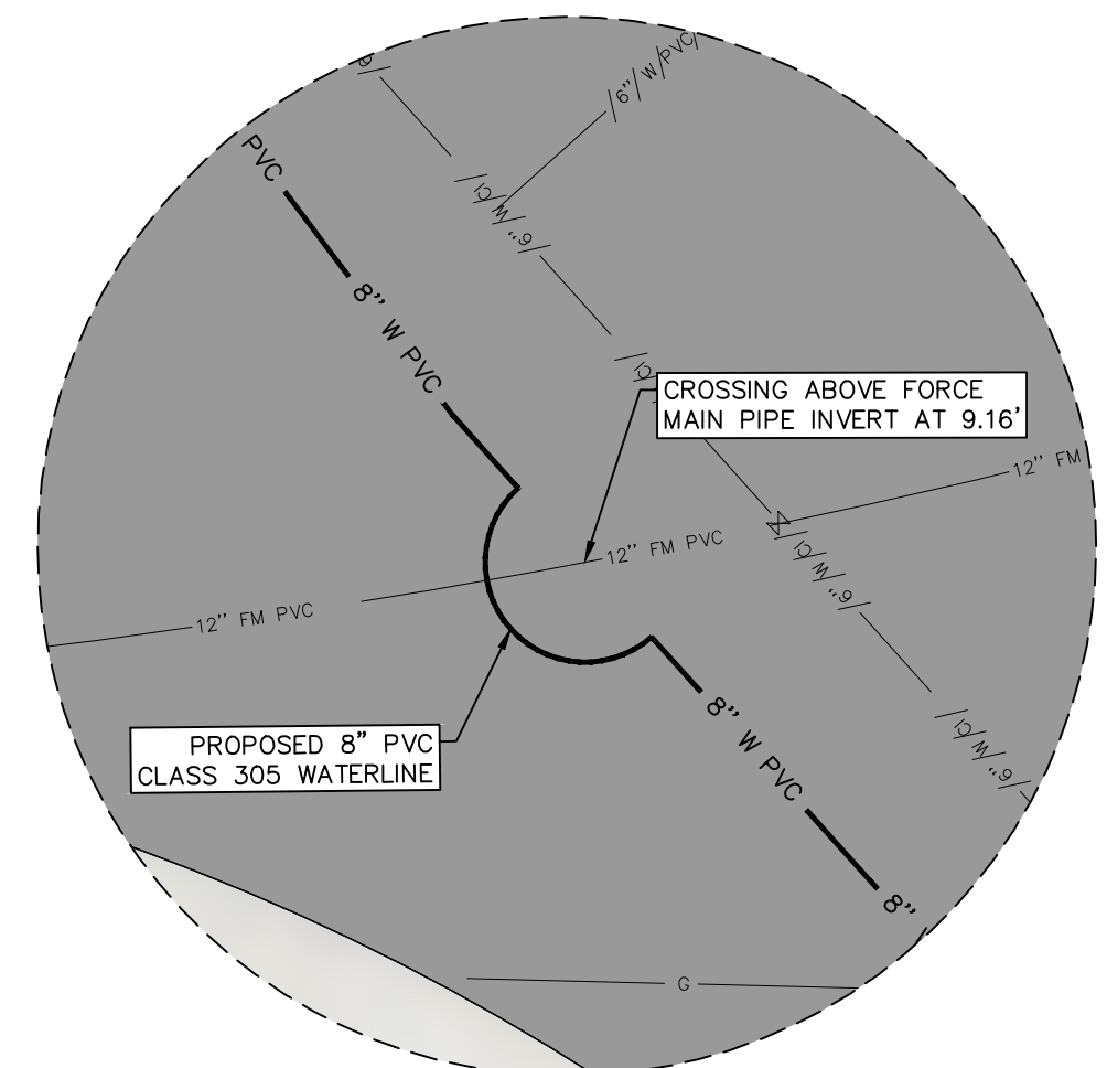
INSET 22 SCALE: 1"=5'
