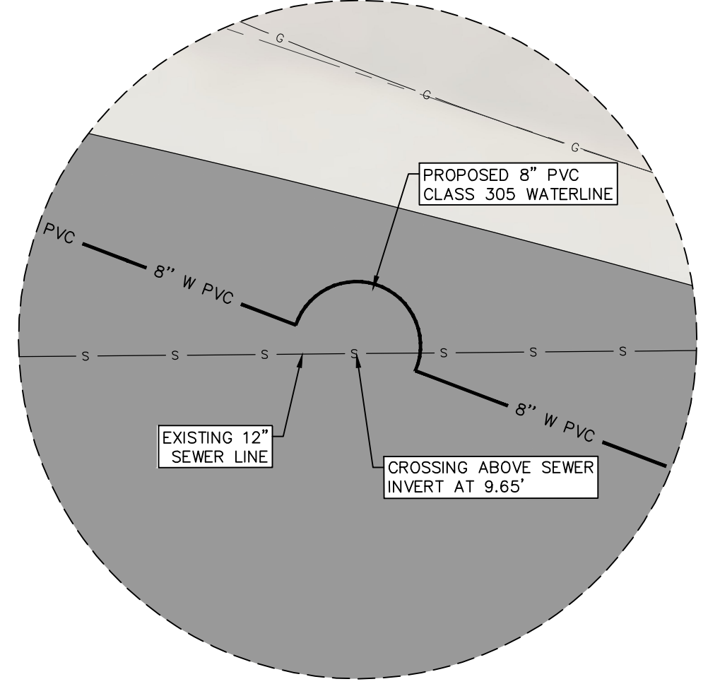
INSET 18 SCALE: 1"=5'
