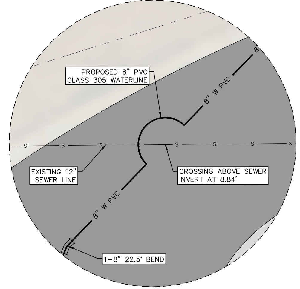
INSET 19 SCALE: 1"=5'
