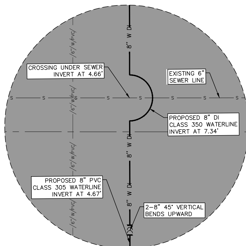
INSET 24 SCALE: 1"=5'
