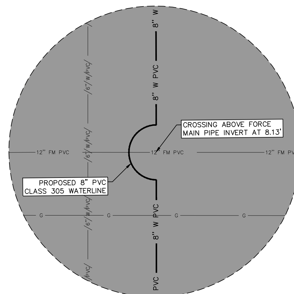
INSET 25 SCALE: 1"=5'
