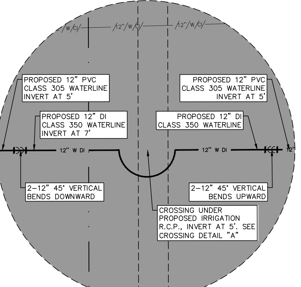
INSET 13 SCALE: 1"=5'
